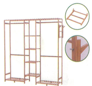
⑨ 取出裤架支架以及裤架档条插入，并且用螺丝固定到侧边支架上
